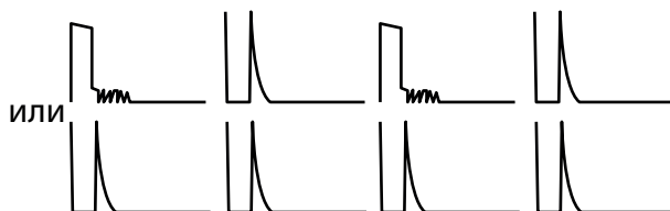
Сигнал управления форсункой
